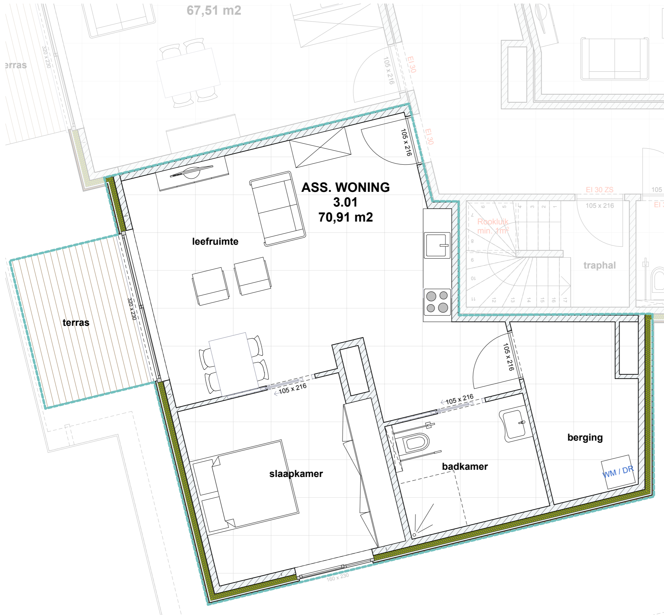
Grondplan - 3e verdieping
