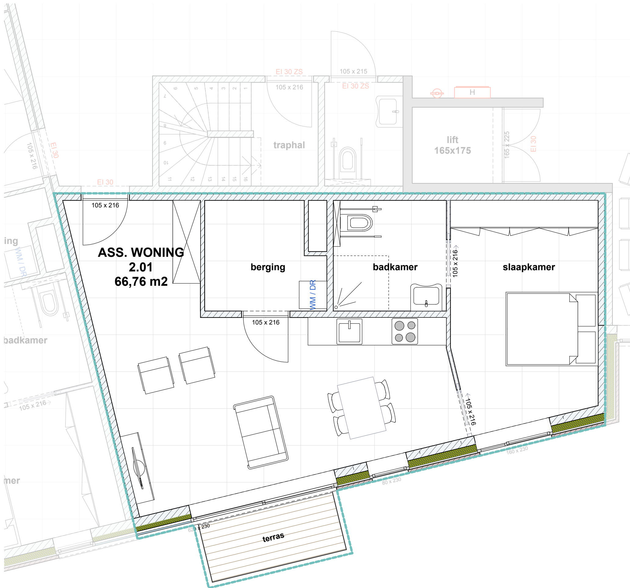
Grondplan - 2e verdieping
